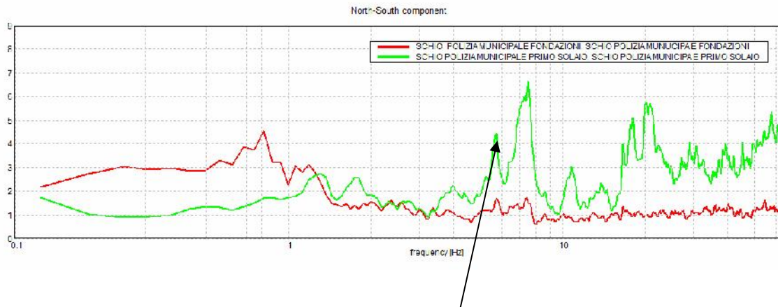
Edificio: Picco Max. at 7.35 Hz
