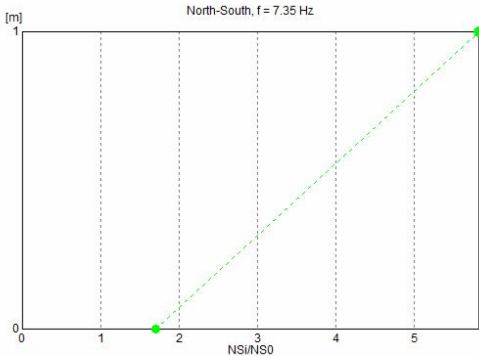
Edificio: Picco Max. at 7.35 Hz
