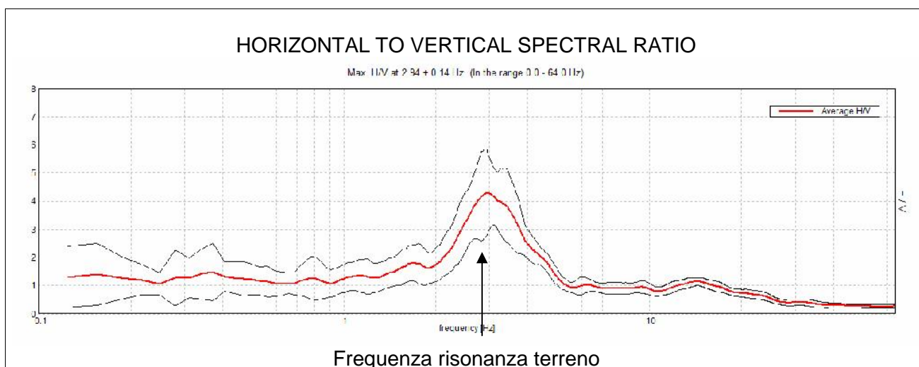
Sito: Picco H/V Terreno Max. H/V at 2.94 Hz
