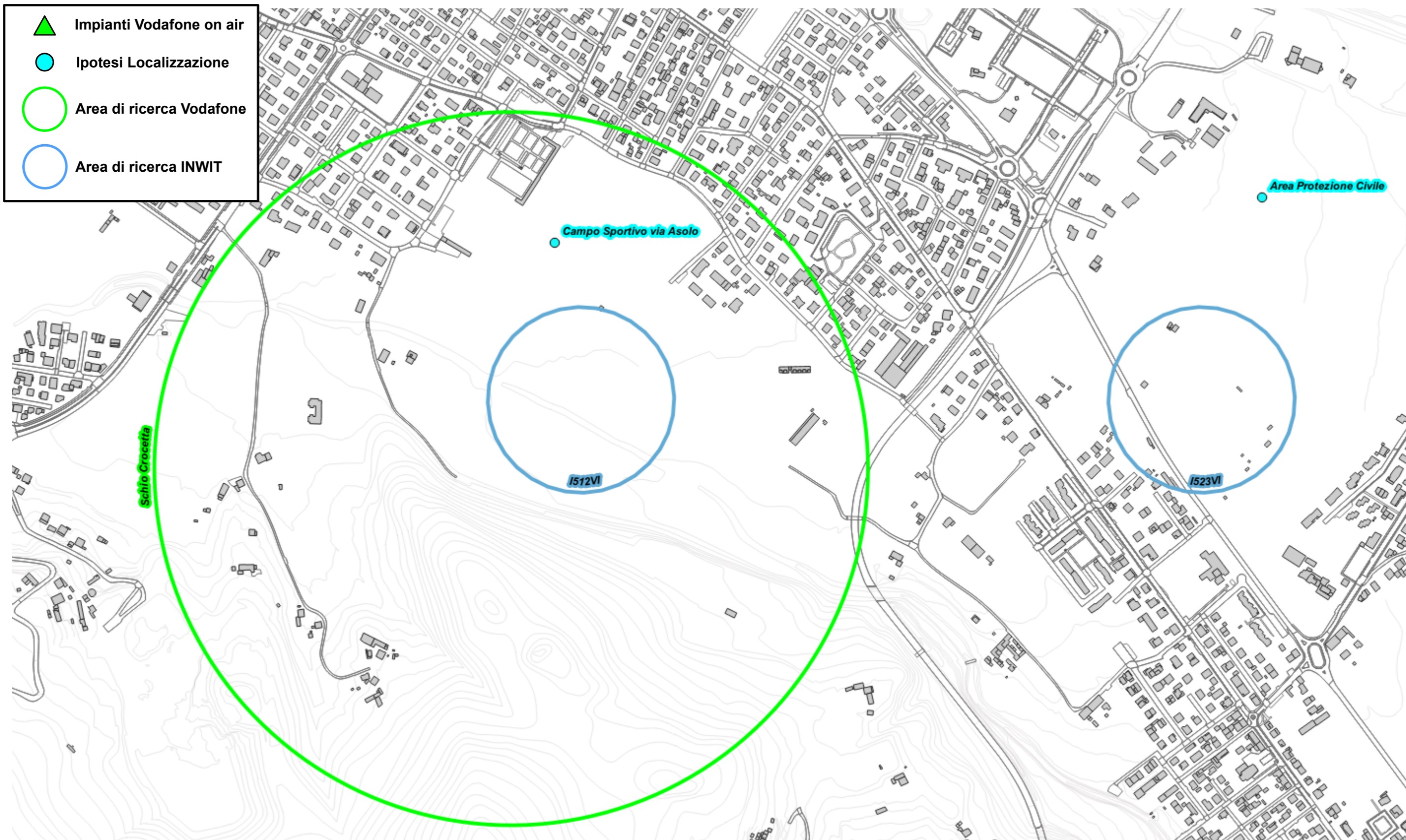
Fig. 26 Dettaglio piano di rete – Gestore VODAFONE
