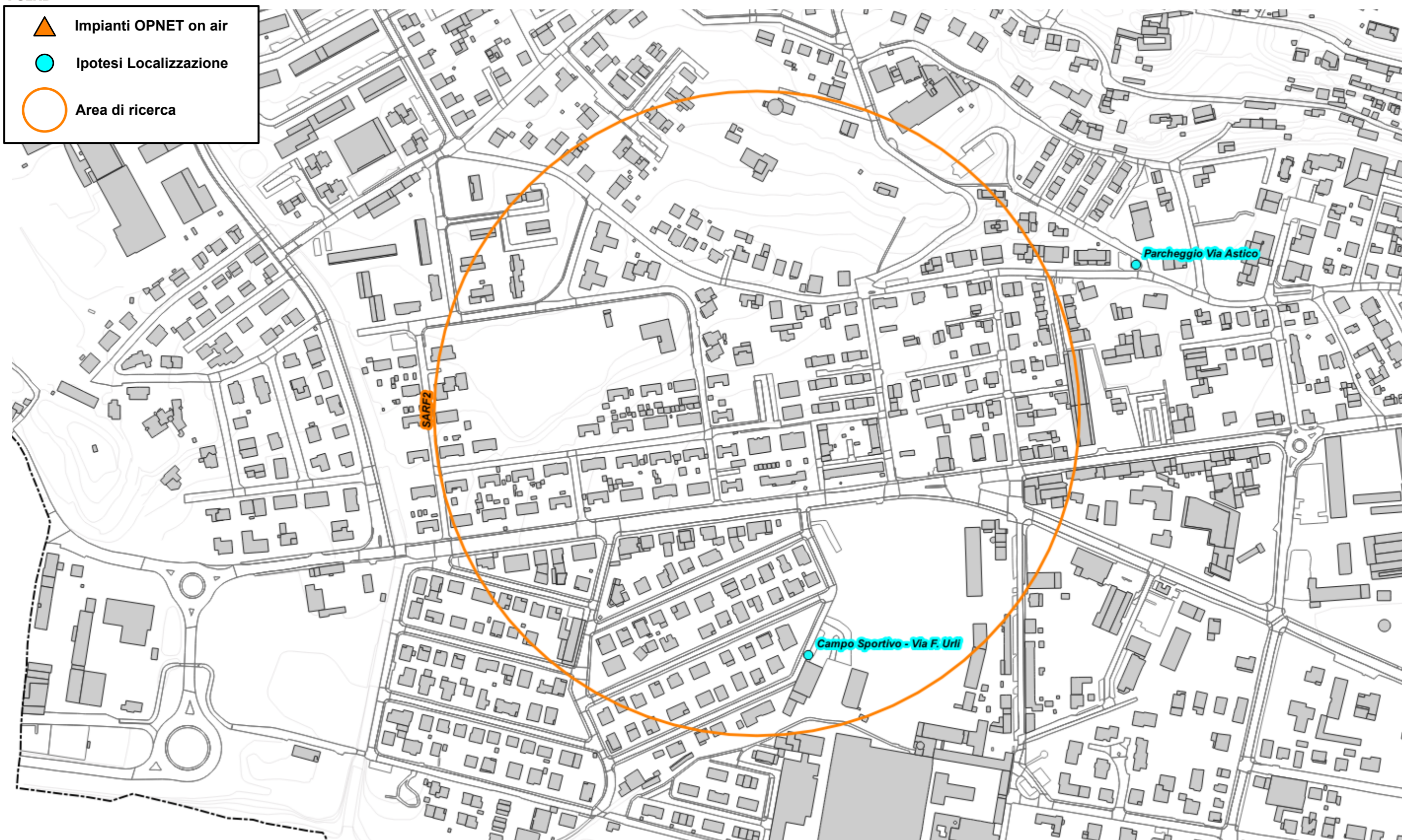
Fig. 42 Dettaglio piano di rete – Gestore OPNET
